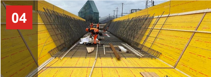
Brückenschalungen
