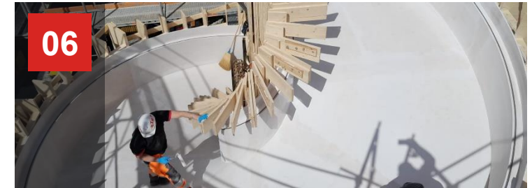
Treppenschalungen
